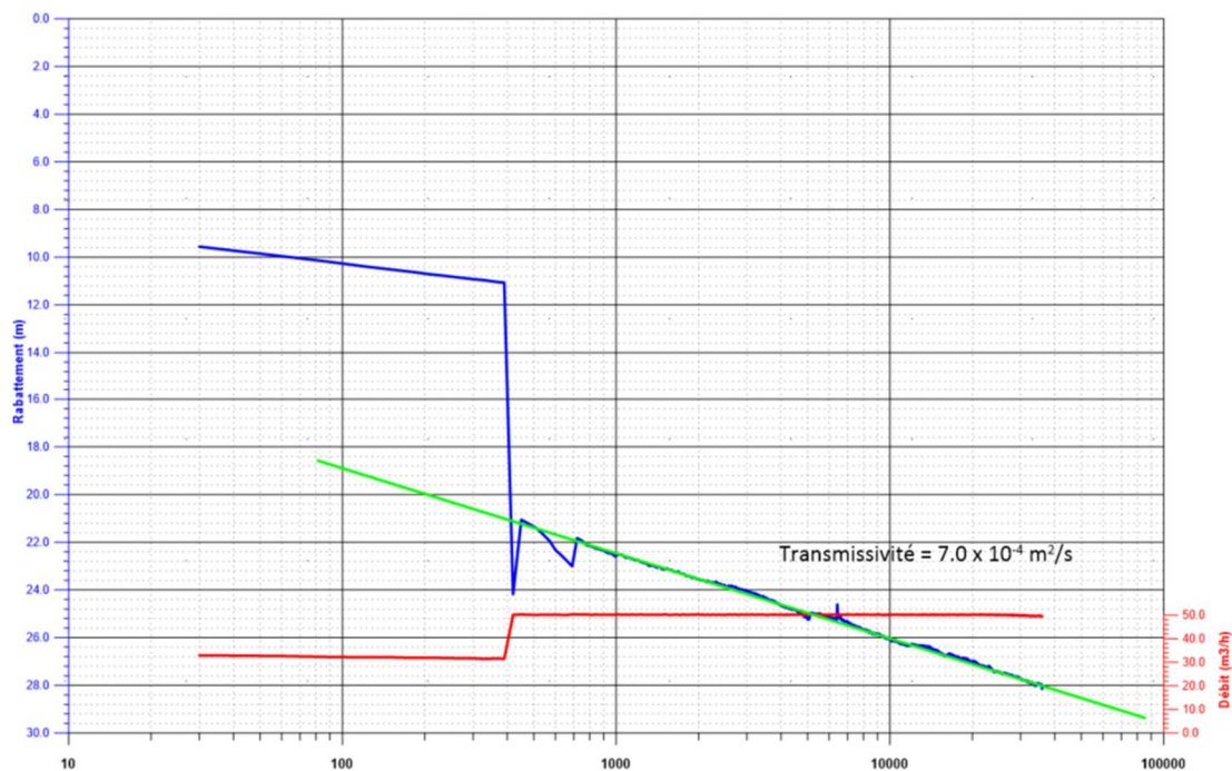
Figure 2 : Estimation de la transmissivité de la formation lors du pompage d'octobre 2023
